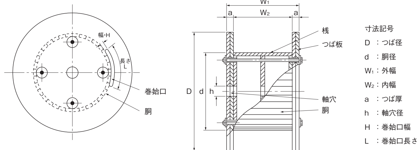
図 一般用木製ドラム構造図の一例
