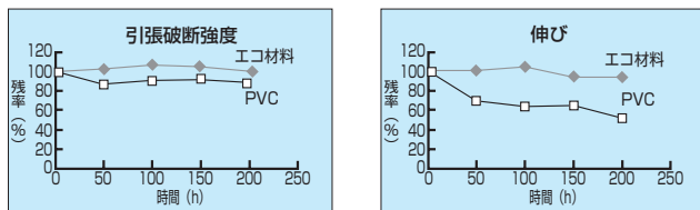
図8 エコ材料とPVCの耐候性の比較 (黄色試料)
