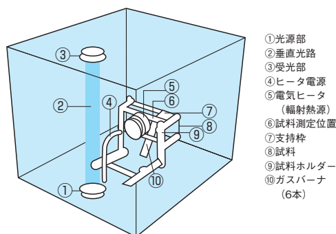
図1 NBSスモークチャンバ (ASTM E 662)
