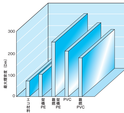
図2 各種材料の発煙性 (ASTM F 662)
