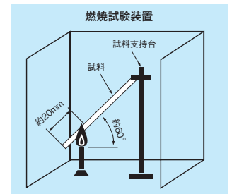
図7 60度傾斜試験
