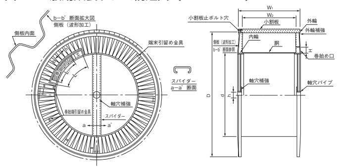
図1 一般用鉄製ドラム構造図 (F11~F15)
