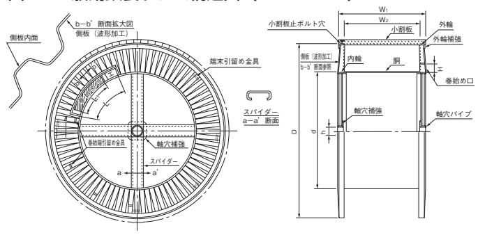
図2 一般用鉄製ドラム構造図 (F16~F18)
