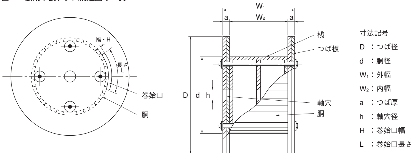
図 一般用木製ドラム構造図の一例
